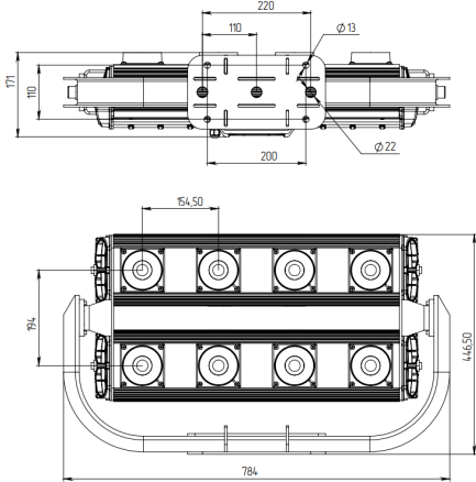
Рисунок 2. Габаритный чертеж
