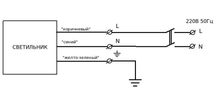
Рисунок 1. Электрическая схема подключения.
